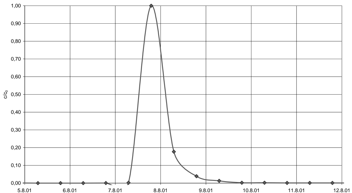
Abb. 3: Normalisierte Durchbruchskurve ( c/c_0 ) des Tracertests im August 2001. Das Maximum entspricht einer Konzentration von 8274 grünen Mikrosphären, die Wiederfindungsrate 5,8 %. Punkte an der Kurve geben den Beprobungszeitpunkt wieder. Zugabe des Tracers am 5.8.2001 um 8:14 Uhr.
