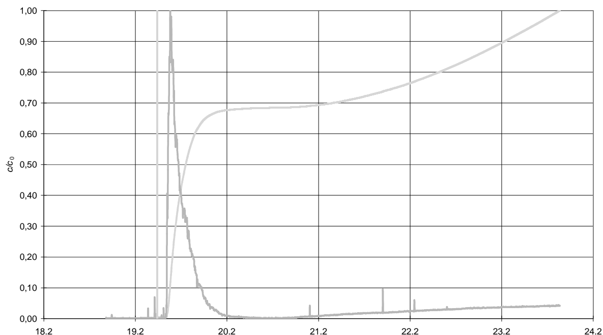
Abb. 4: Normalisierte Durchbruchskurve ( c/c_0 ) des Tracertests mit Uranin im Februar 2002. Das Maximum entspricht einer Konzentration von 300 \mu\text{g L}^{-1} , die Wiederfindungsrate 2,6 %. Vertikale Linie nach dem 19.2.: Injektion des Tracers.
